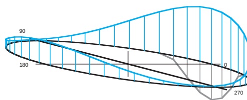
KA040XP0 带有径向载荷100 lbs、轴向载荷100lbs、 扭矩载荷30Inch-lbs
