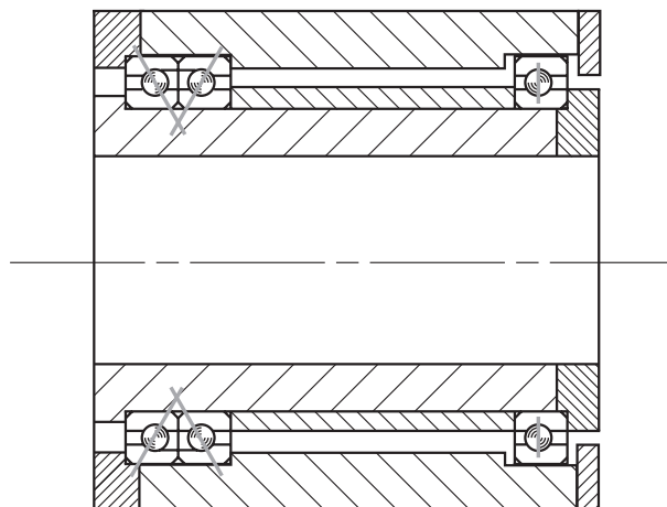
图 3-27B 面对面
