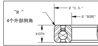
开式轴承
