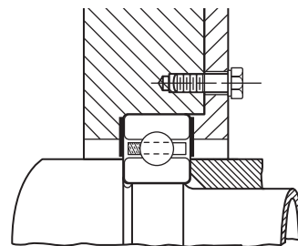
图 2-9 精密垫片防尘盖
