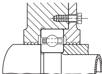
图 2-8 环形沟
