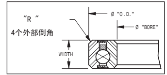
密封轴承
