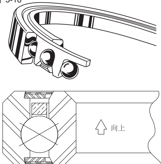
图示为正确的轴承方向
