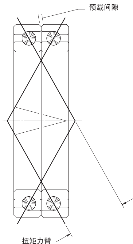
图 3-4 面对面（DF 型）
