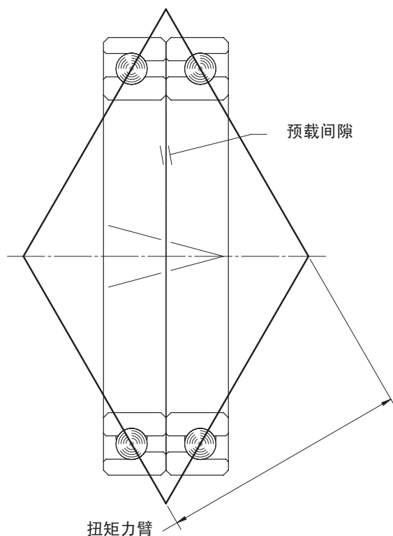
图 3-3 背对背（DB 型）
