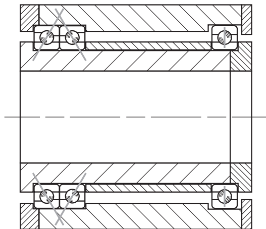
图 3-27B 面对面
