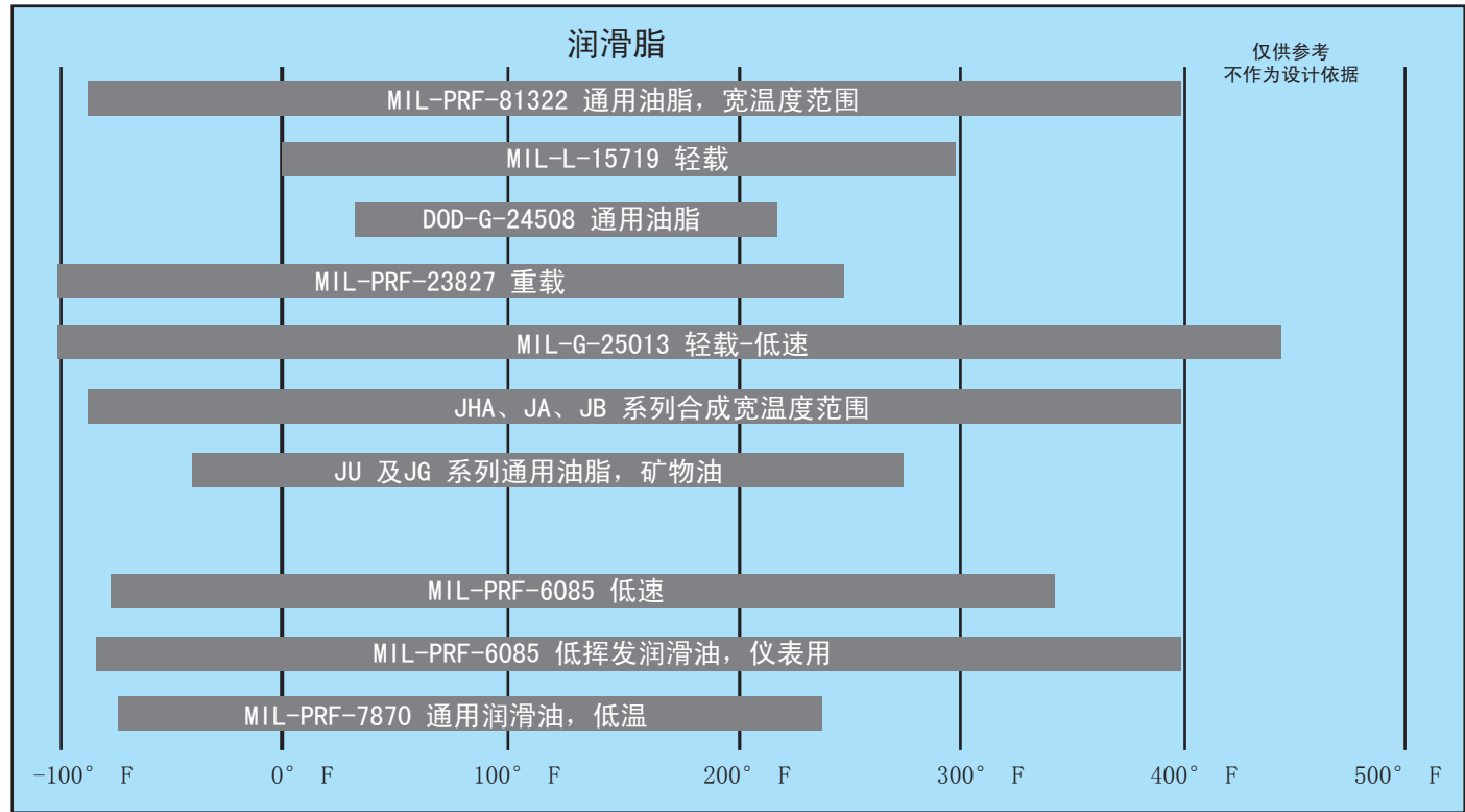
图 5-2 润滑剂温度范围
